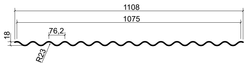
Secțiune A-A
