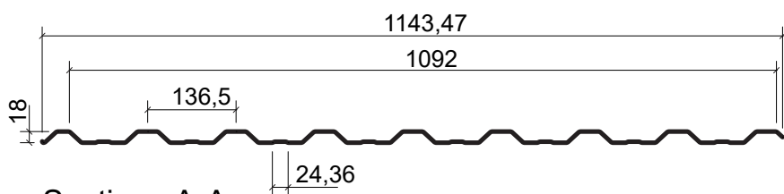
Sețiune A-A
